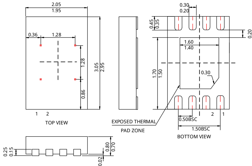
DFN2030-8L 封装外形图
