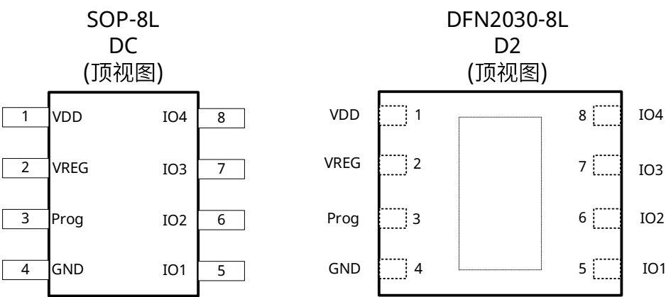
图 2 SOP-8L 封装顶视图(左)&DFN2030-8L 封装顶视图(右)
