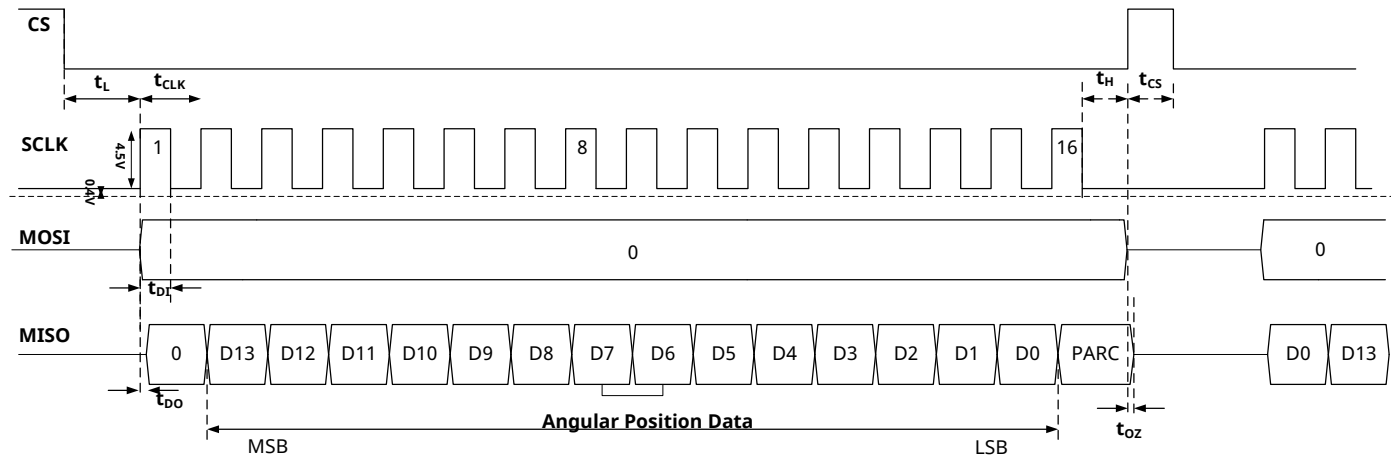
图 11 SPI 角度读取模式图
